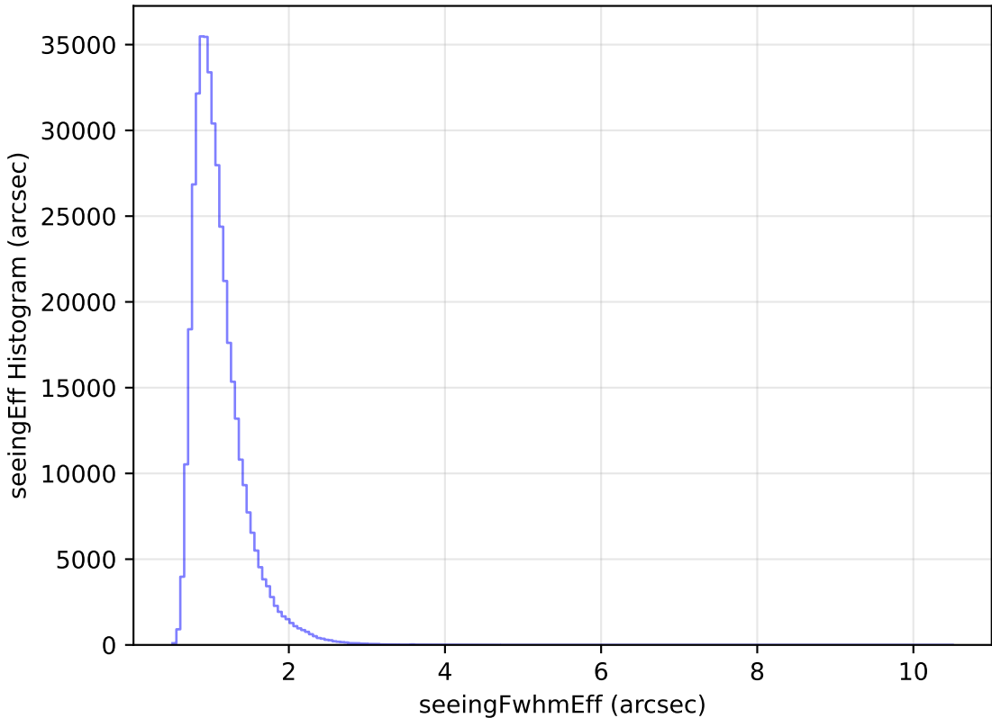
weather_cloudso18v3.4_10yrs WFD y band: seeingEff Histogram
