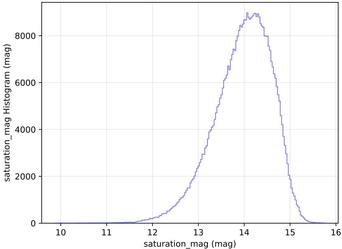
weather_cloudso18v3.4_10yrs WFD z band: saturation_mag Histogram
