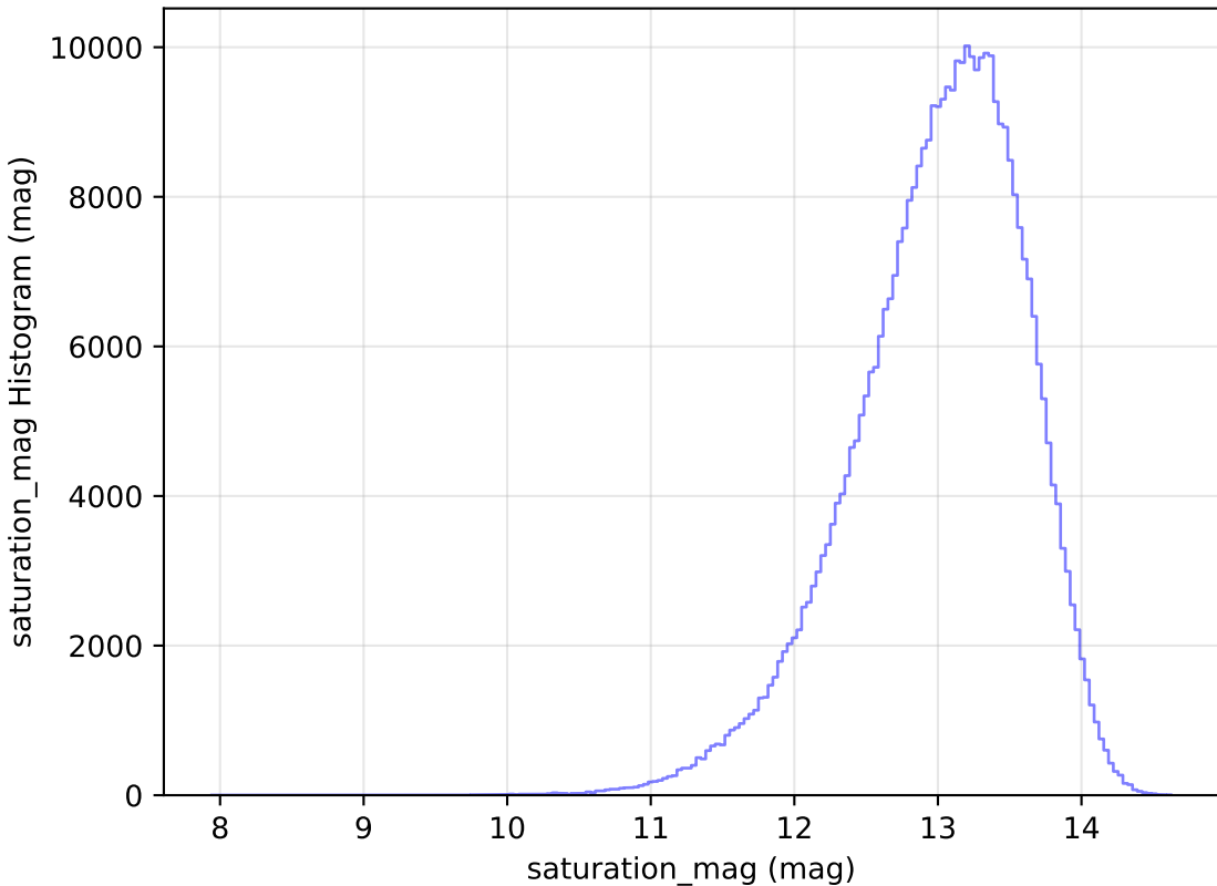
weather_cloudso18v3.4_10yrs WFD y band: saturation_mag Histogram
