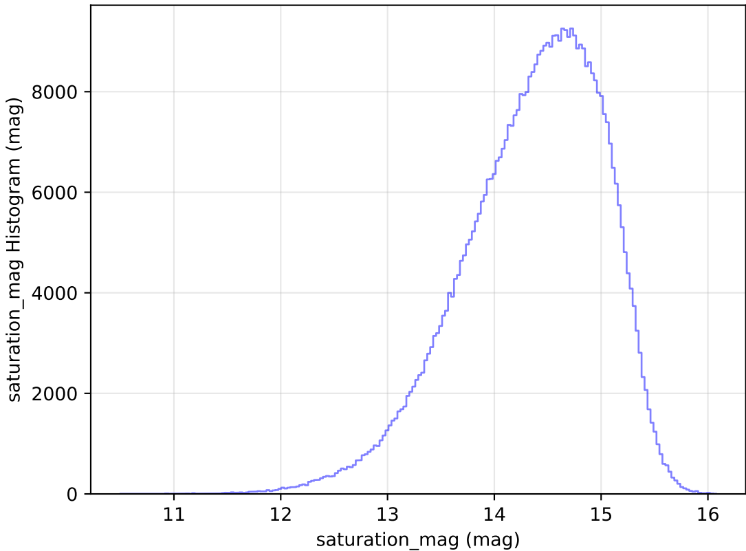
weather_cloudso18v3.4_10yrs WFD i band: saturation_mag Histogram
