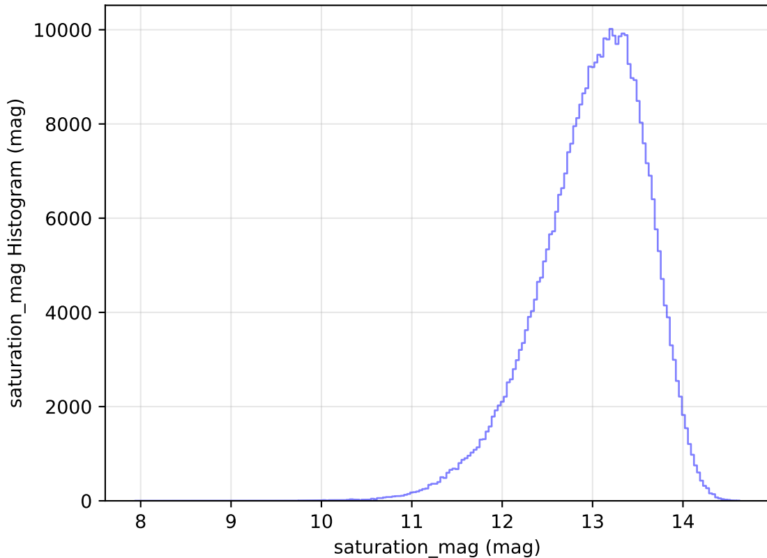
weather_cloudso18v3.4_10yrs All sky y band: saturation_mag Histogram
