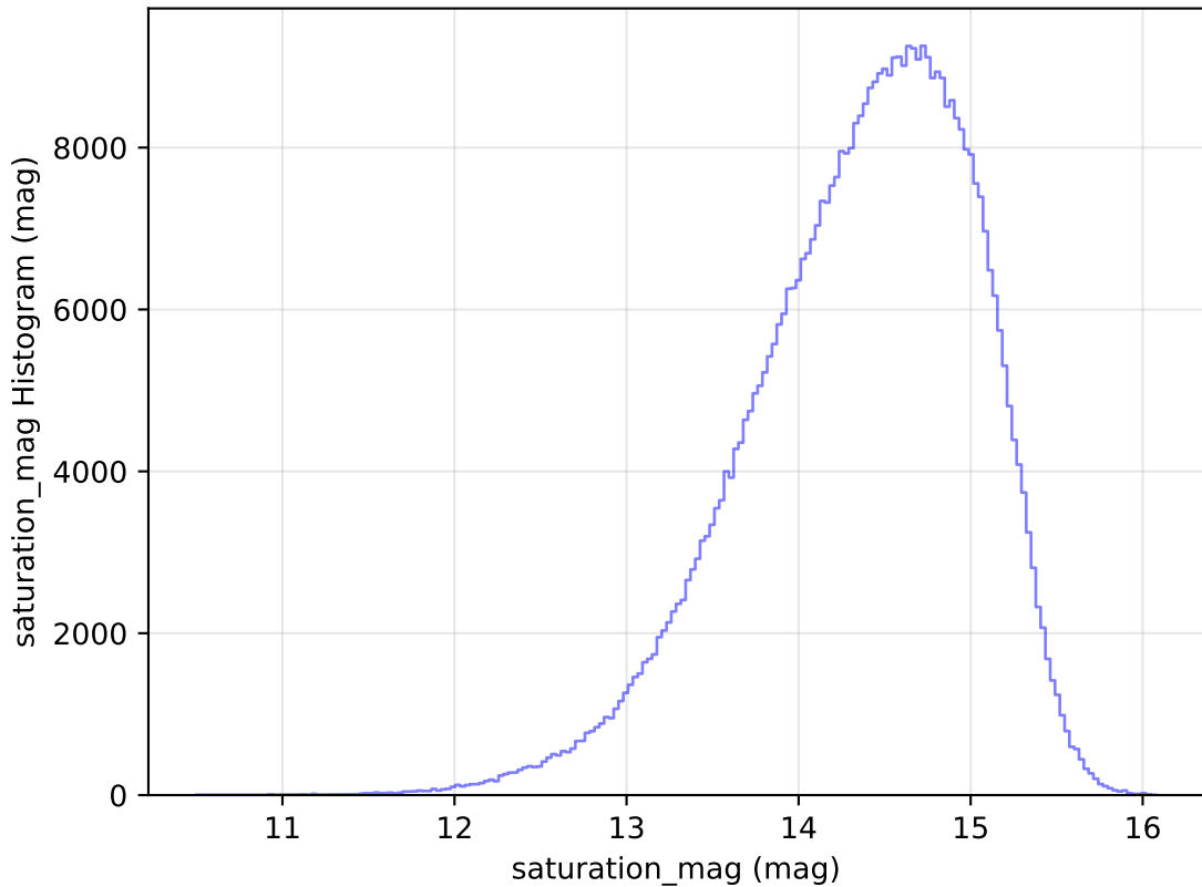
weather_cloudso18v3.4_10yrs All sky i band: saturation_mag Histogram
