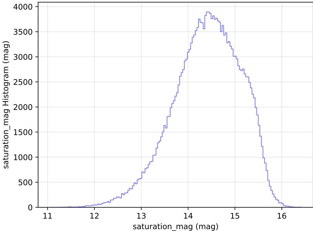
weather_cloudso18v3.4_10yrs All sky g band: saturation_mag Histogram
