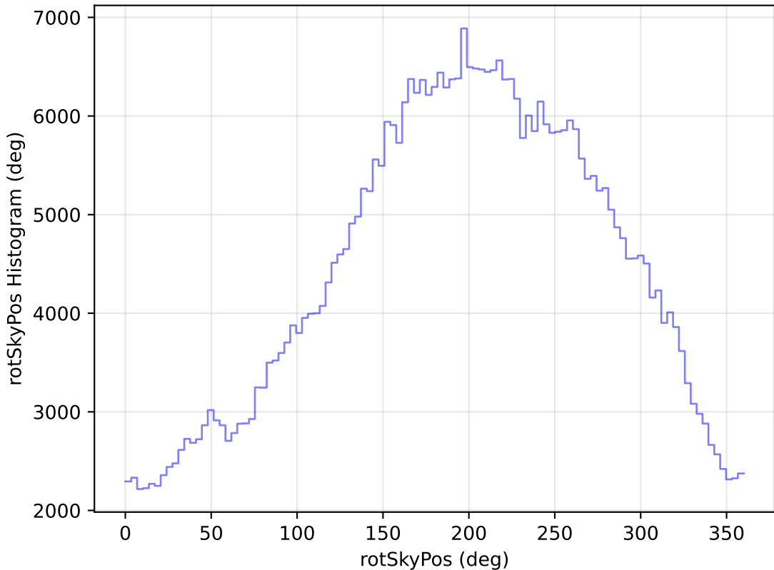
weather_cloudso18v3.4_10yrs WFD z band: rotSkyPos Histogram
