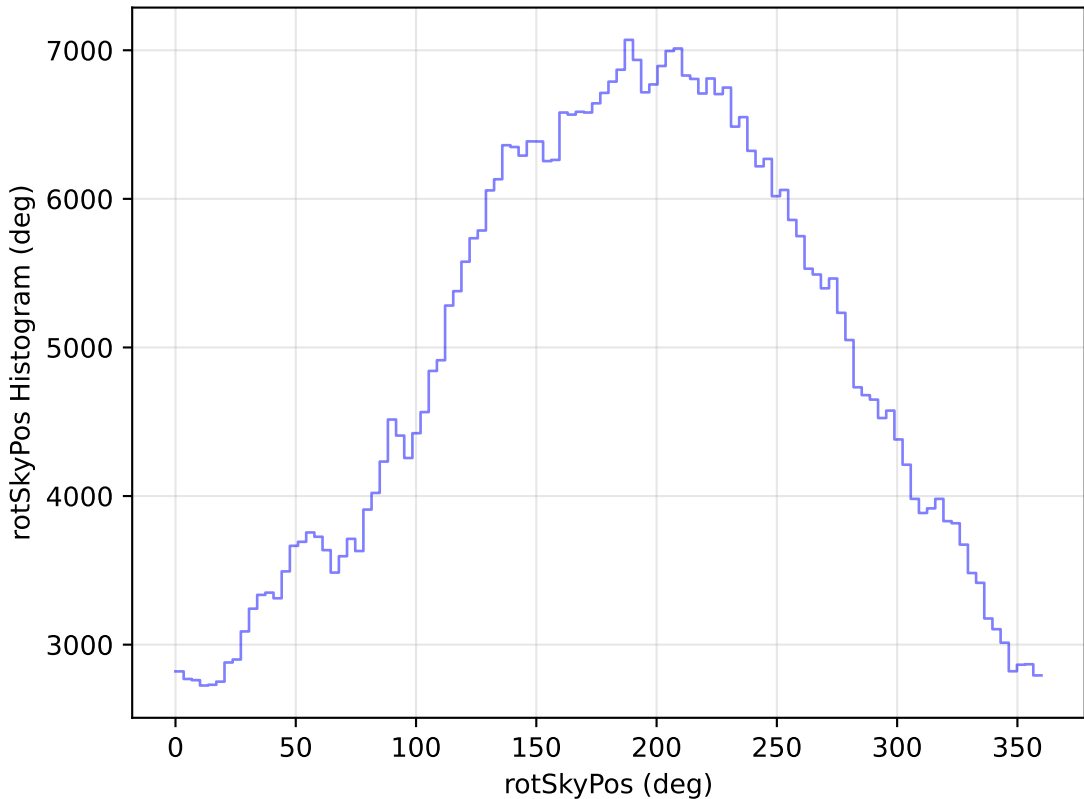
weather_cloudso18v3.4_10yrs WFD r band: rotSkyPos Histogram
