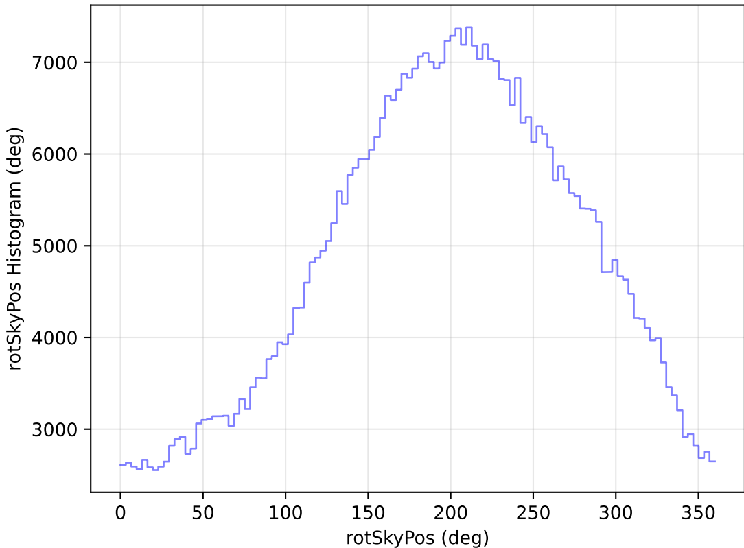
weather_cloudso18v3.4_10yrs WFD i band: rotSkyPos Histogram
