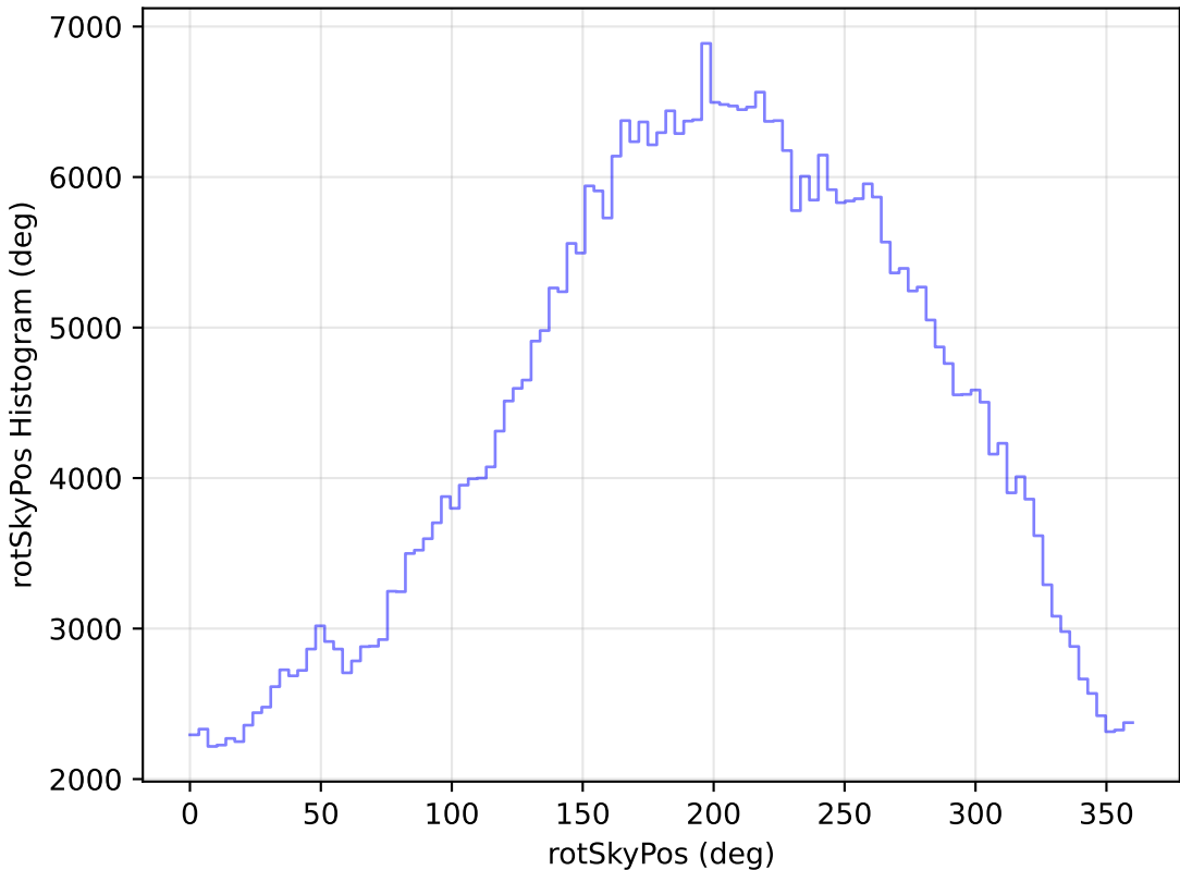
weather_cloudso18v3.4_10yrs All sky z band: rotSkyPos Histogram
