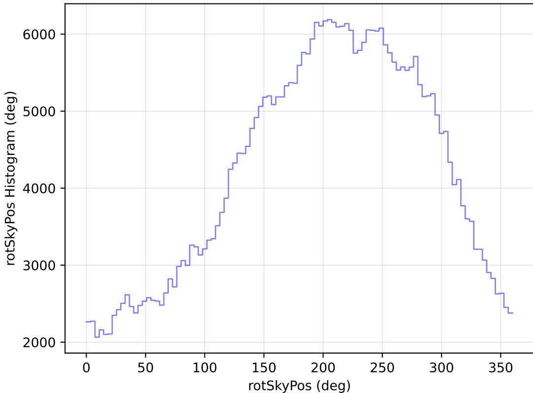
weather_cloudso18v3.4_10yrs All sky y band: rotSkyPos Histogram
