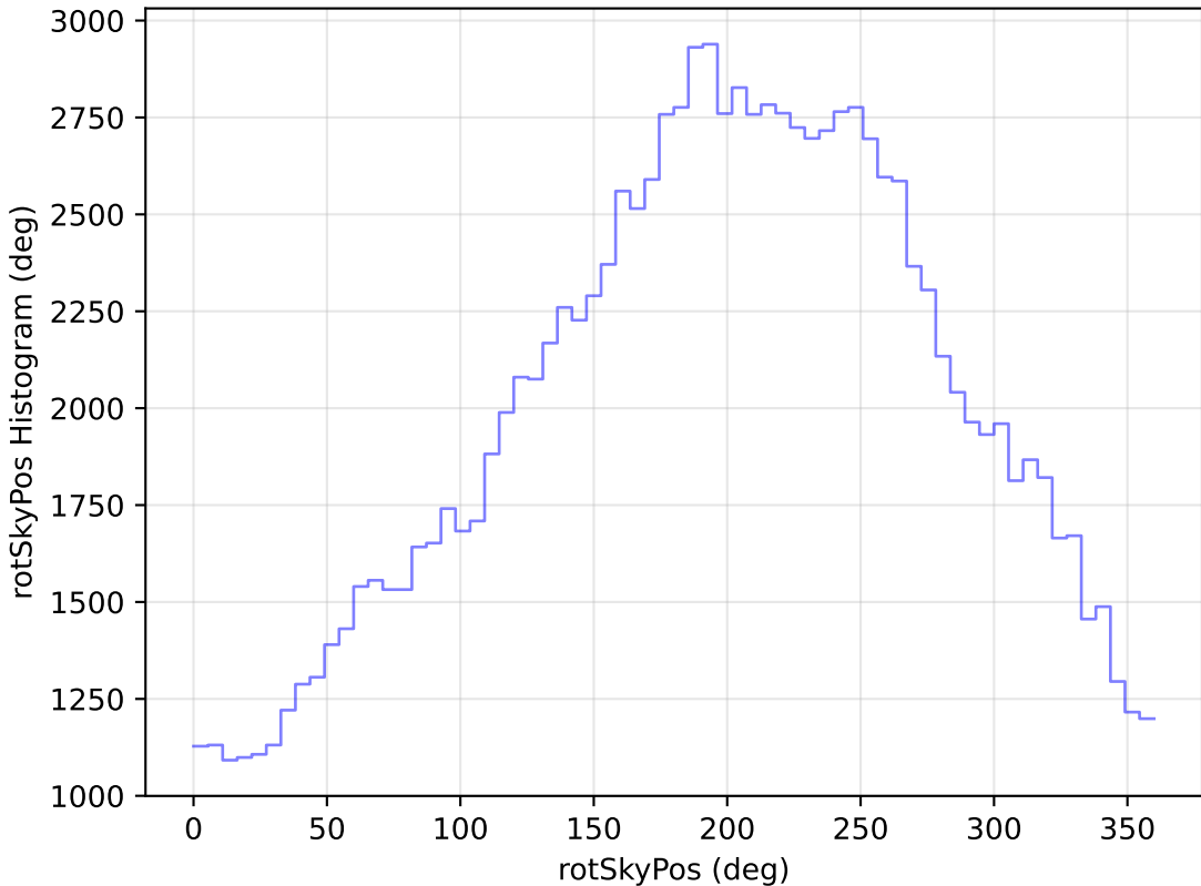
weather_cloudso18v3.4_10yrs All sky u band: rotSkyPos Histogram
