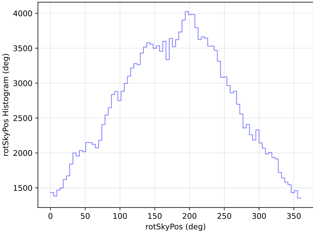
weather_cloudso18v3.4_10yrs All sky g band: rotSkyPos Histogram
