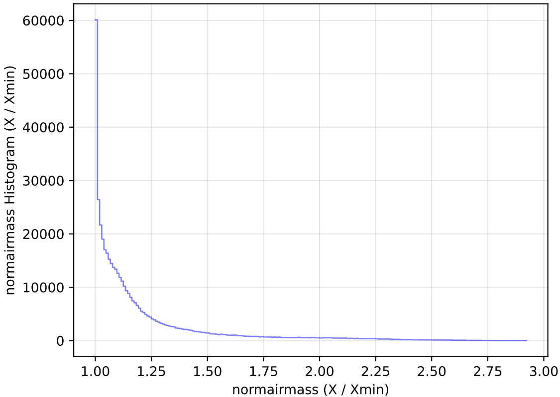
weather_cloudso18v3.4_10yrs WFD z band: normairmass Histogram
