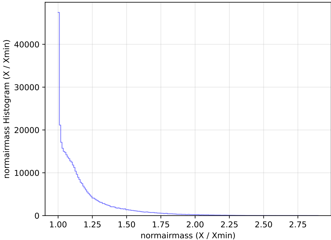
weather_cloudso18v3.4_10yrs WFD y band: normairmass Histogram
