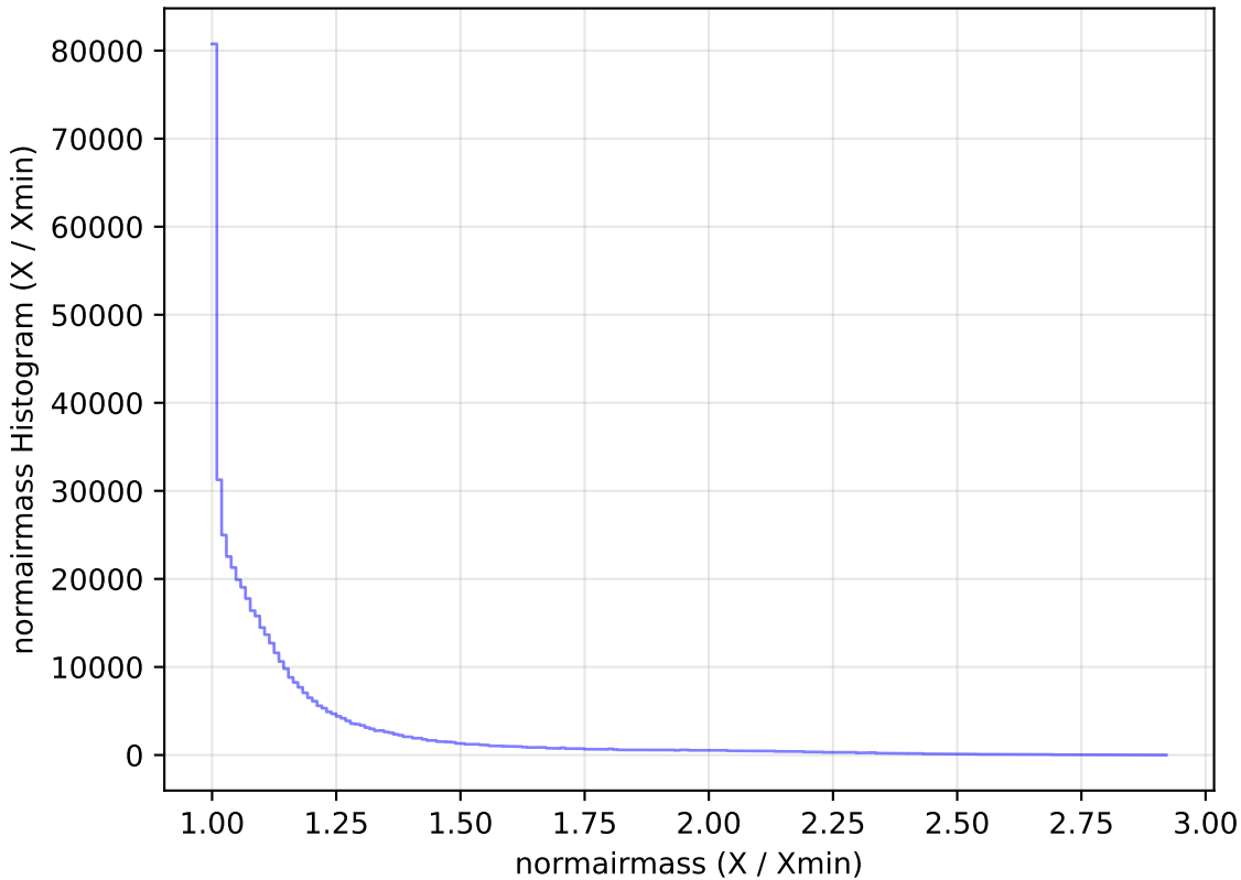
weather_cloudso18v3.4_10yrs WFD i band: normairmass Histogram
