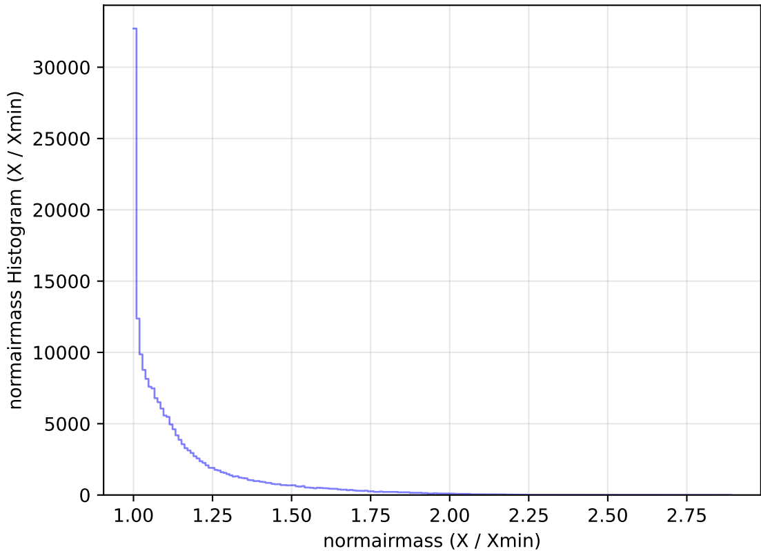
weather_cloudso18v3.4_10yrs WFD g band: normairmass Histogram
