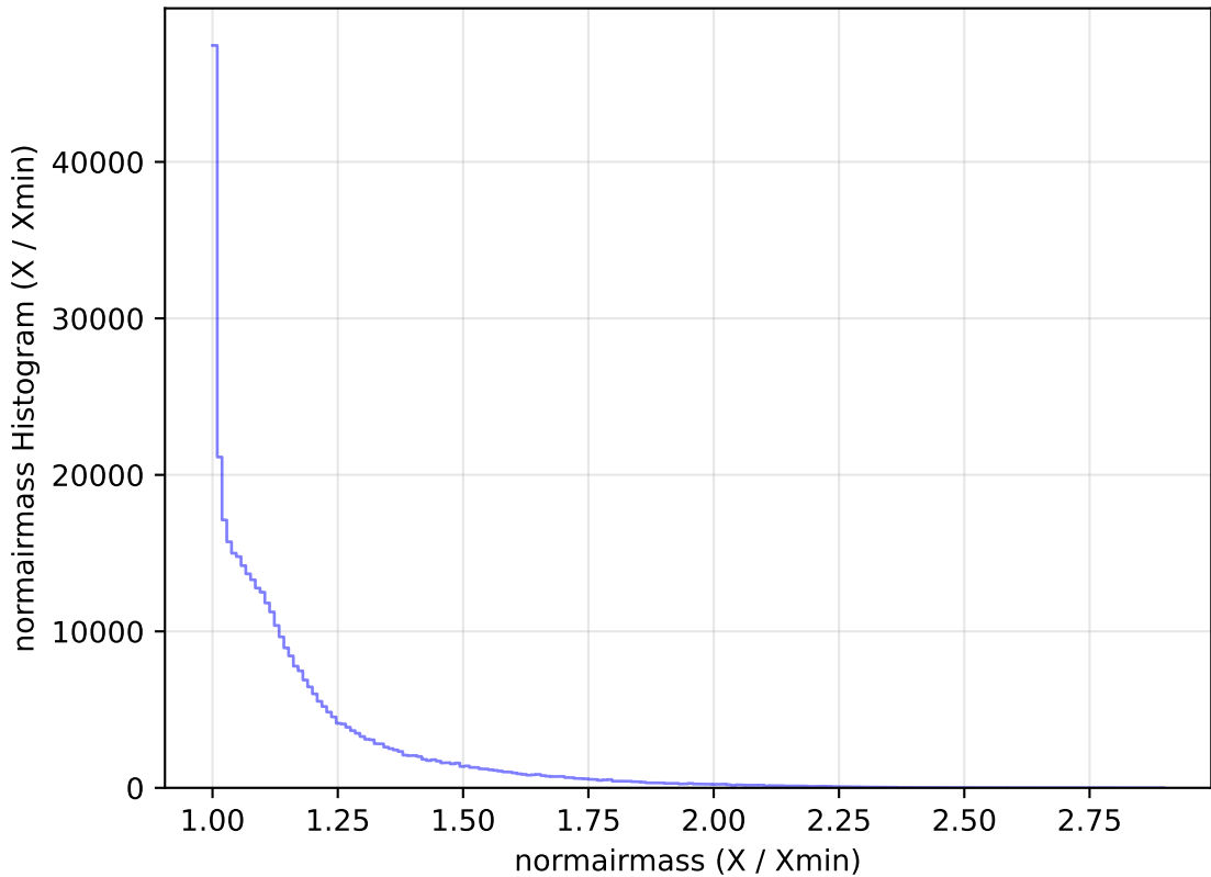
weather_cloudso18v3.4_10yrs All sky y band: normairmass Histogram
