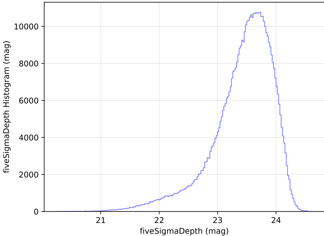
weather_cloudso18v3.4_10yrs WFD i band: fiveSigmaDepth Histogram
