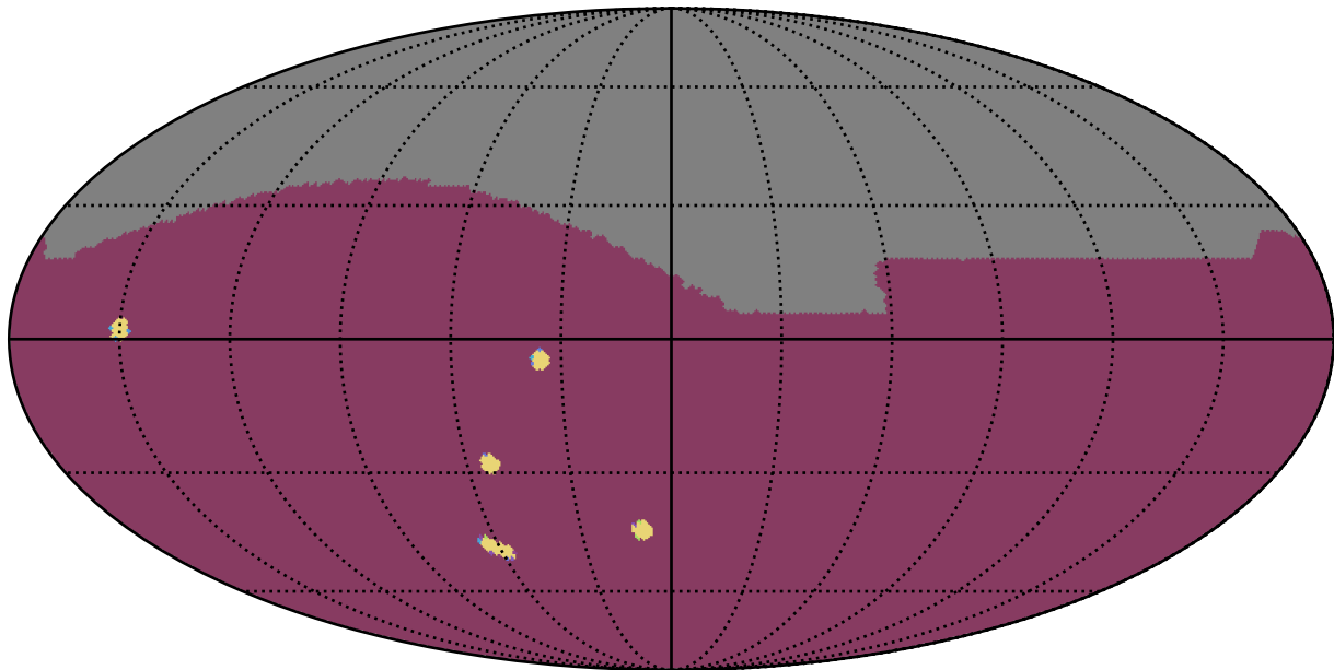
weather_cloudso18v3.4_10yrs All sky: NumberOfQuickRevisits
