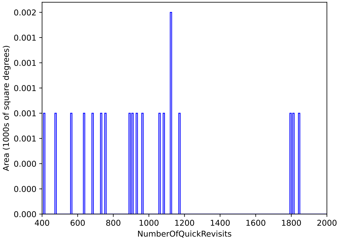
weather_cloudso18v3.4_10yrs All sky: NumberOfQuickRevisits
