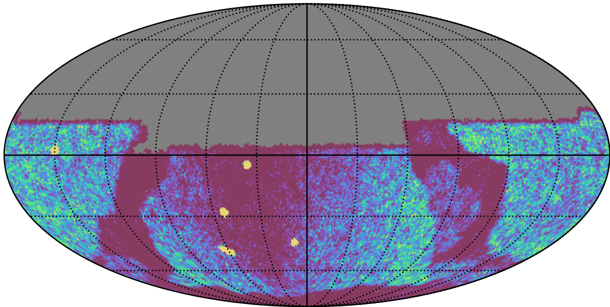
weather_cloudso18v3.4_10yrs Yr 1 y band: NVisits
