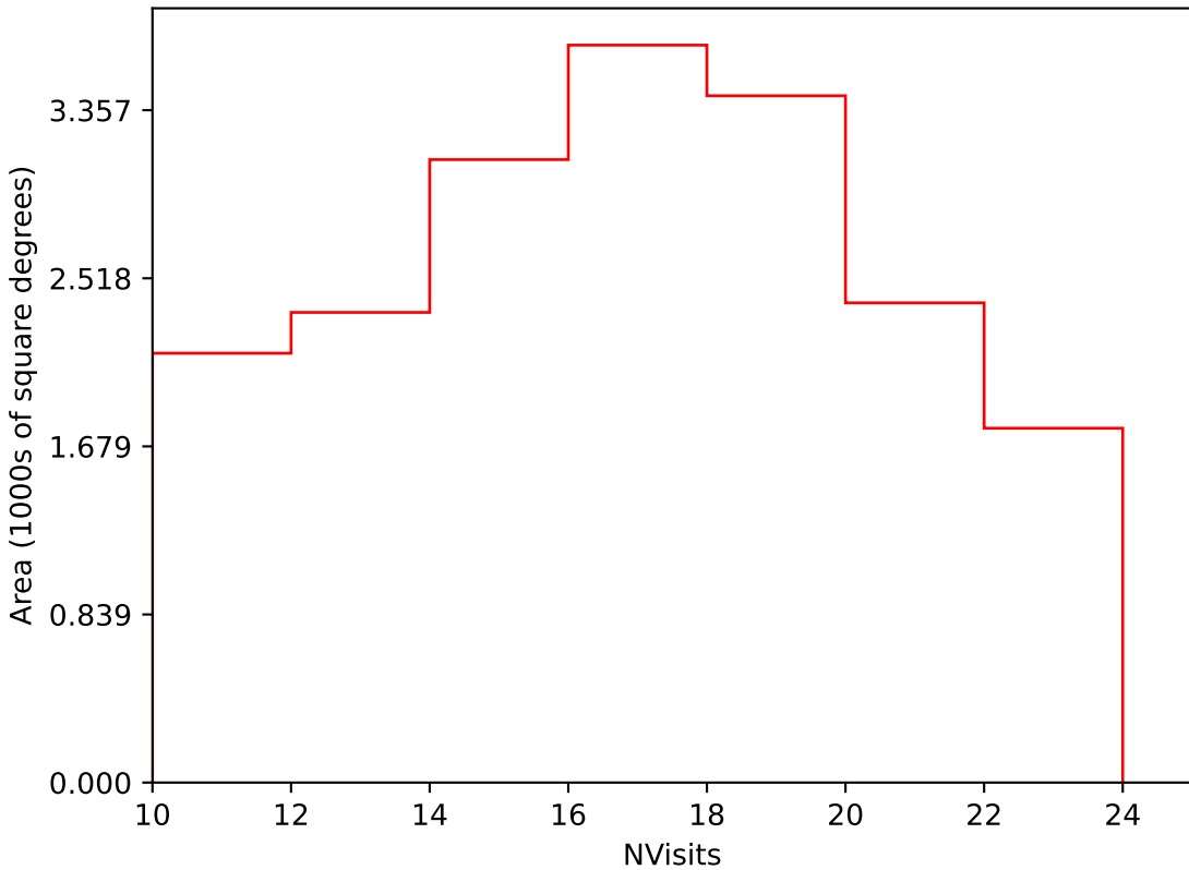
weather_cloudso18v3.4_10yrs Yr 1 i band: NVisits
