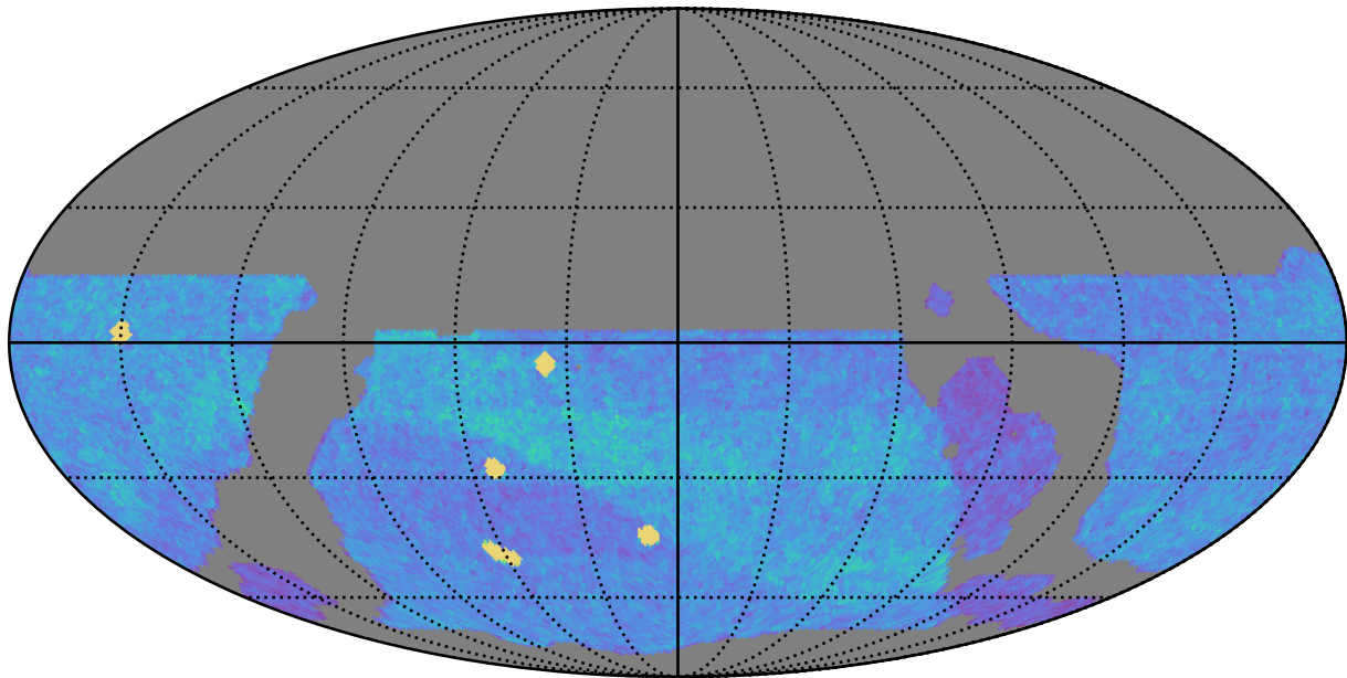
weather_cloudso18v3.4_10yrs WFD z band: NVisits
