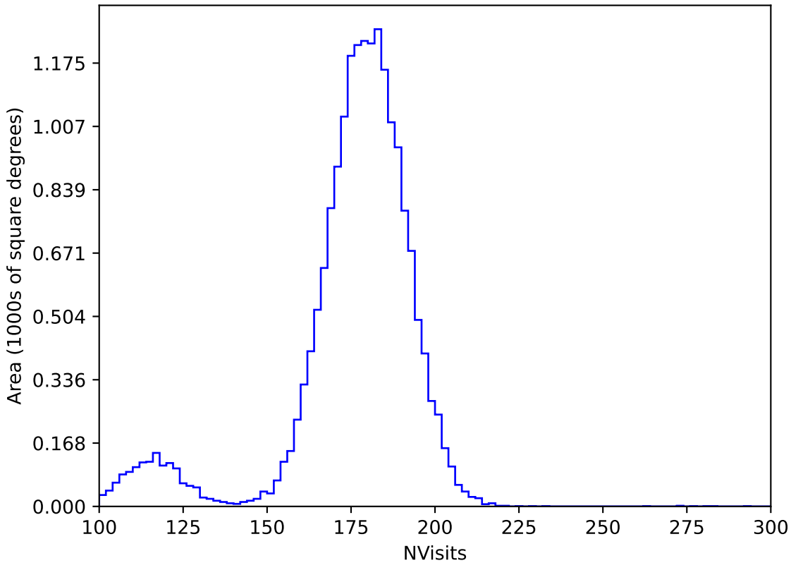
weather_cloudso18v3.4_10yrs WFD y band: NVisits
