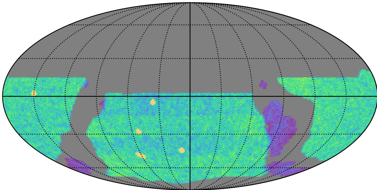
weather_cloudso18v3.4_10yrs WFD u band: NVisits
