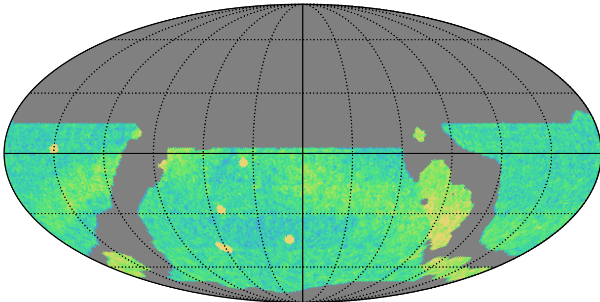
weather_cloudso18v3.4_10yrs WFD r band: NVisits
