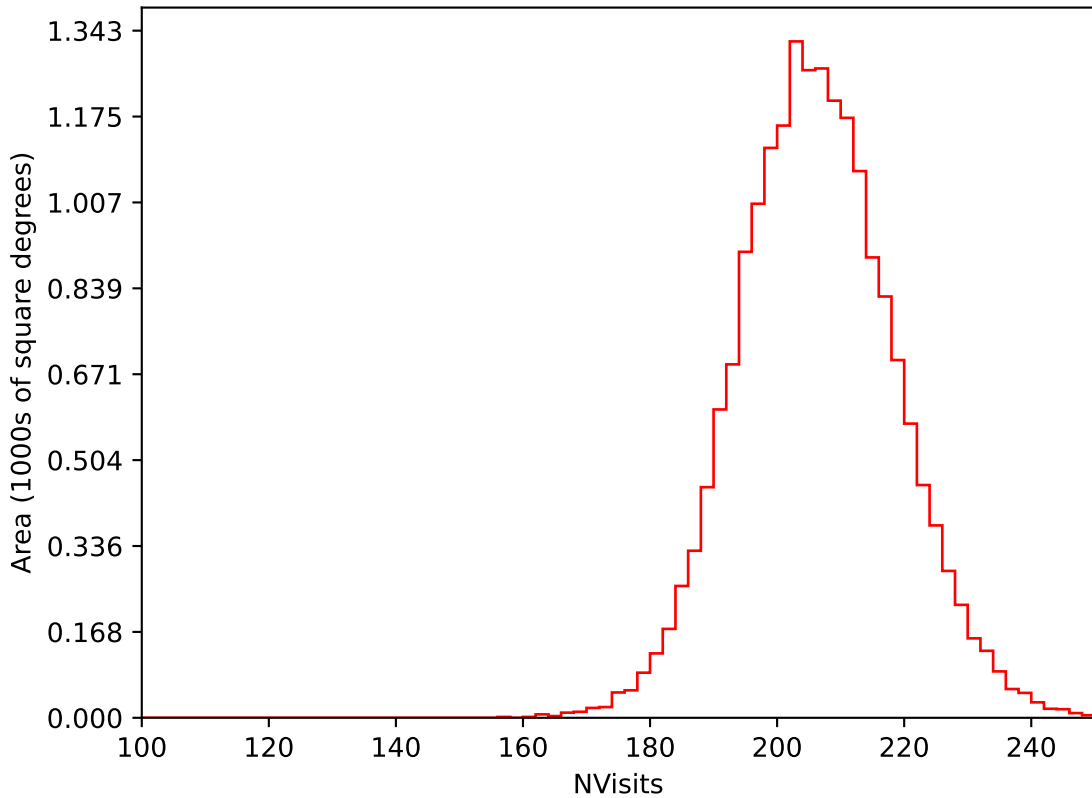
weather_cloudso18v3.4_10yrs WFD i band: NVisits
