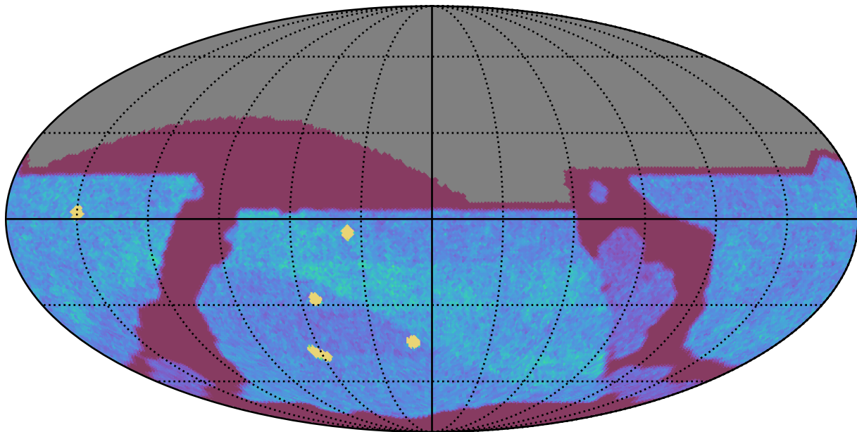
weather_cloudso18v3.4_10yrs All sky z band: NVisits
