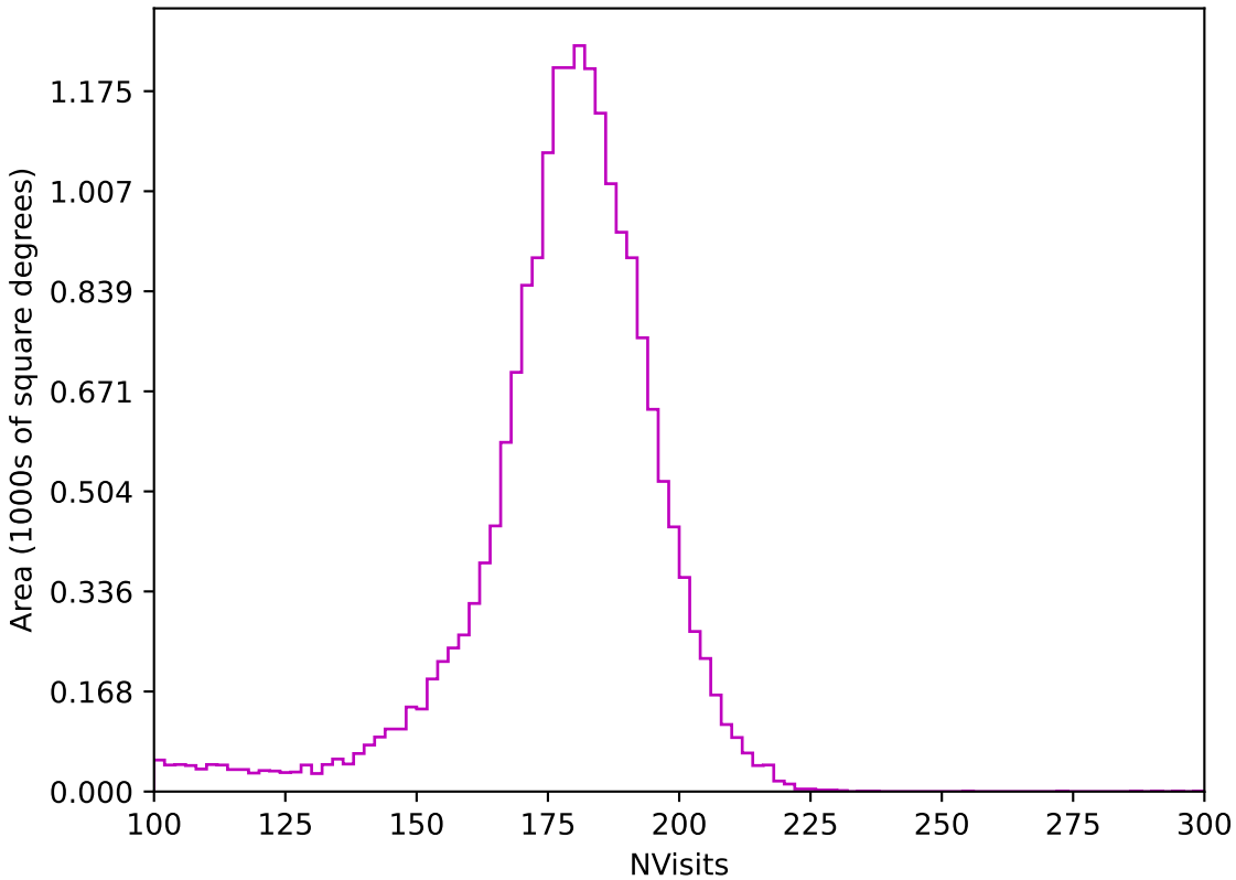
weather_cloudso18v3.4_10yrs All sky z band: NVisits
