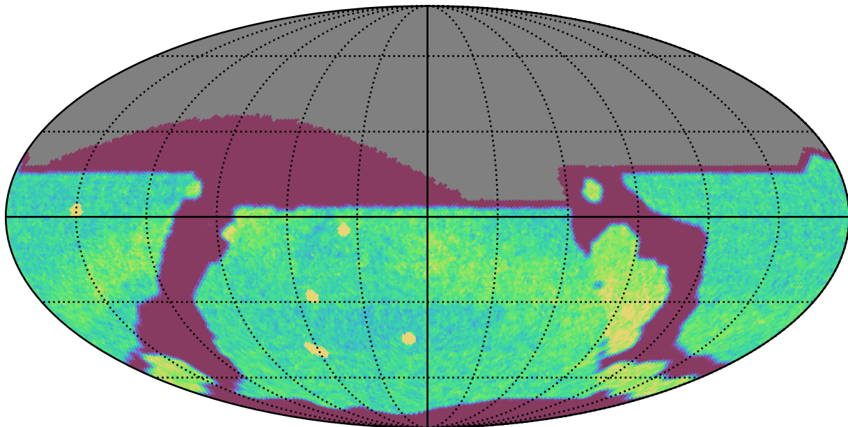
weather_cloudso18v3.4_10yrs All sky r band: NVisits
