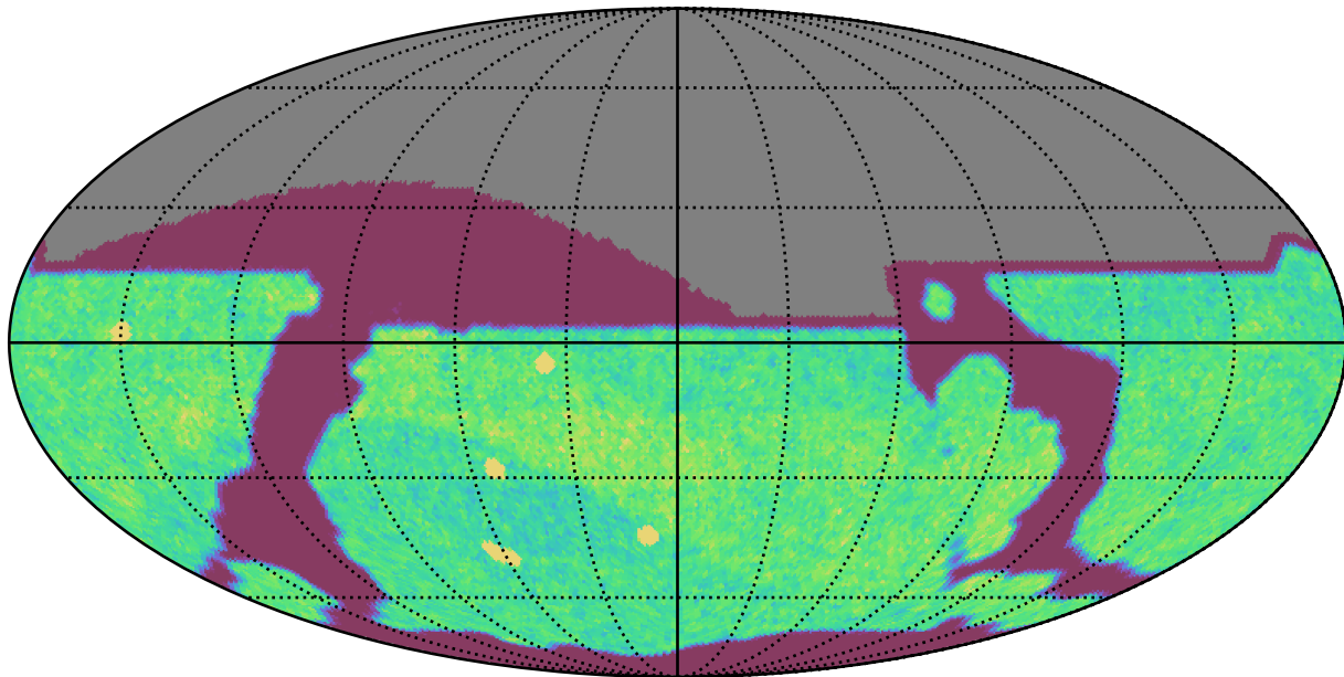
weather_cloudso18v3.4_10yrs All sky i band: NVisits
