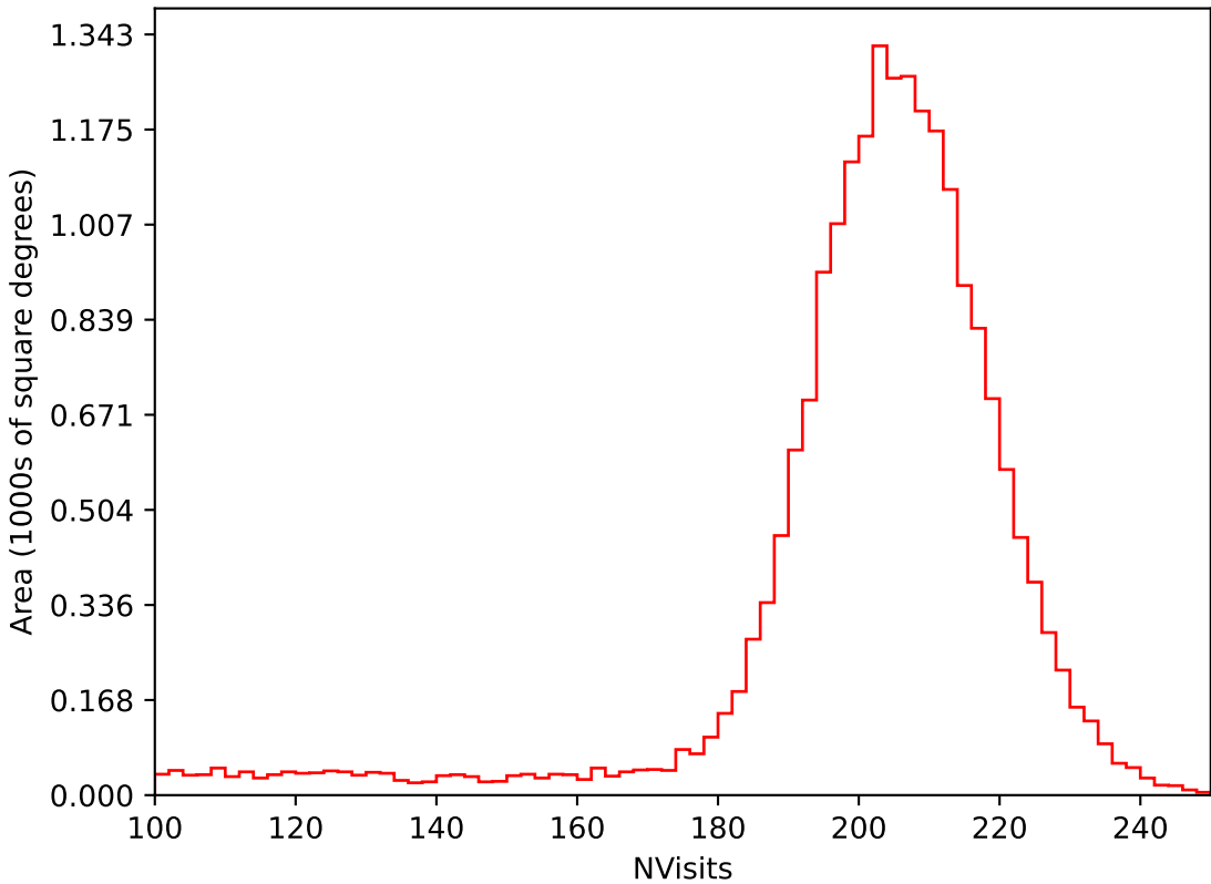
weather_cloudso18v3.4_10yrs All sky i band: NVisits
