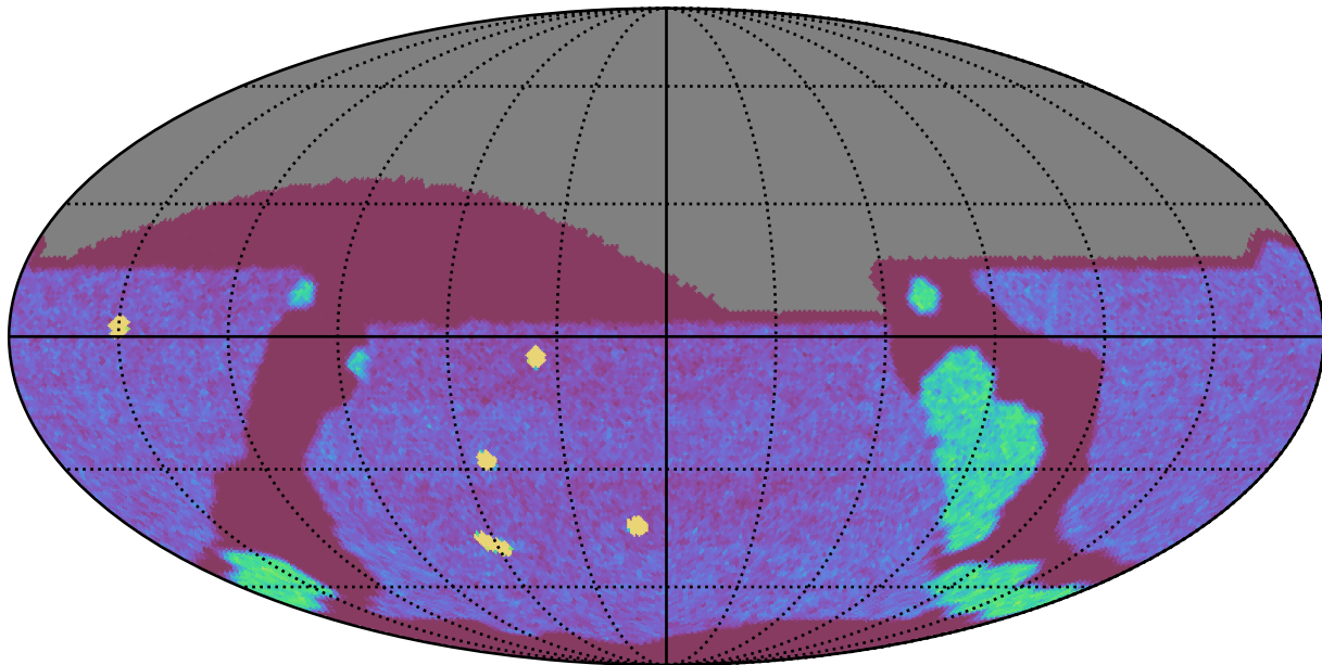
weather_cloudso18v3.4_10yrs All sky g band: NVisits
