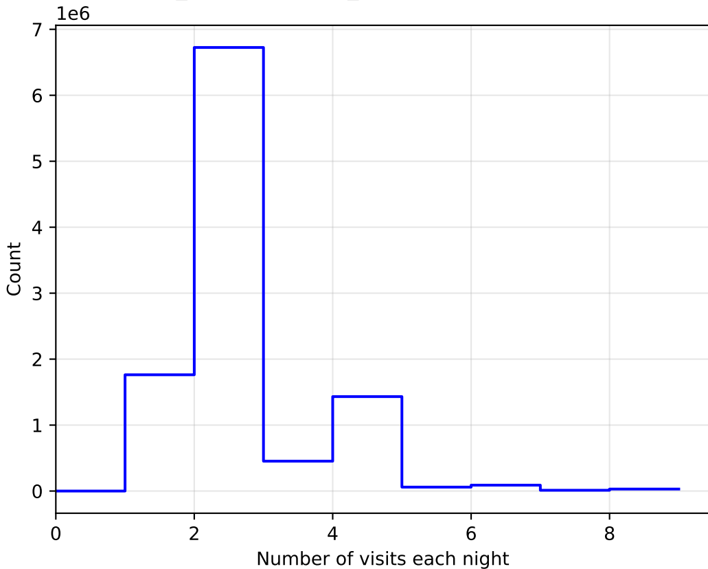
weather_cloudso18v3.4_10yrs All sky: NVisitsPerNight
