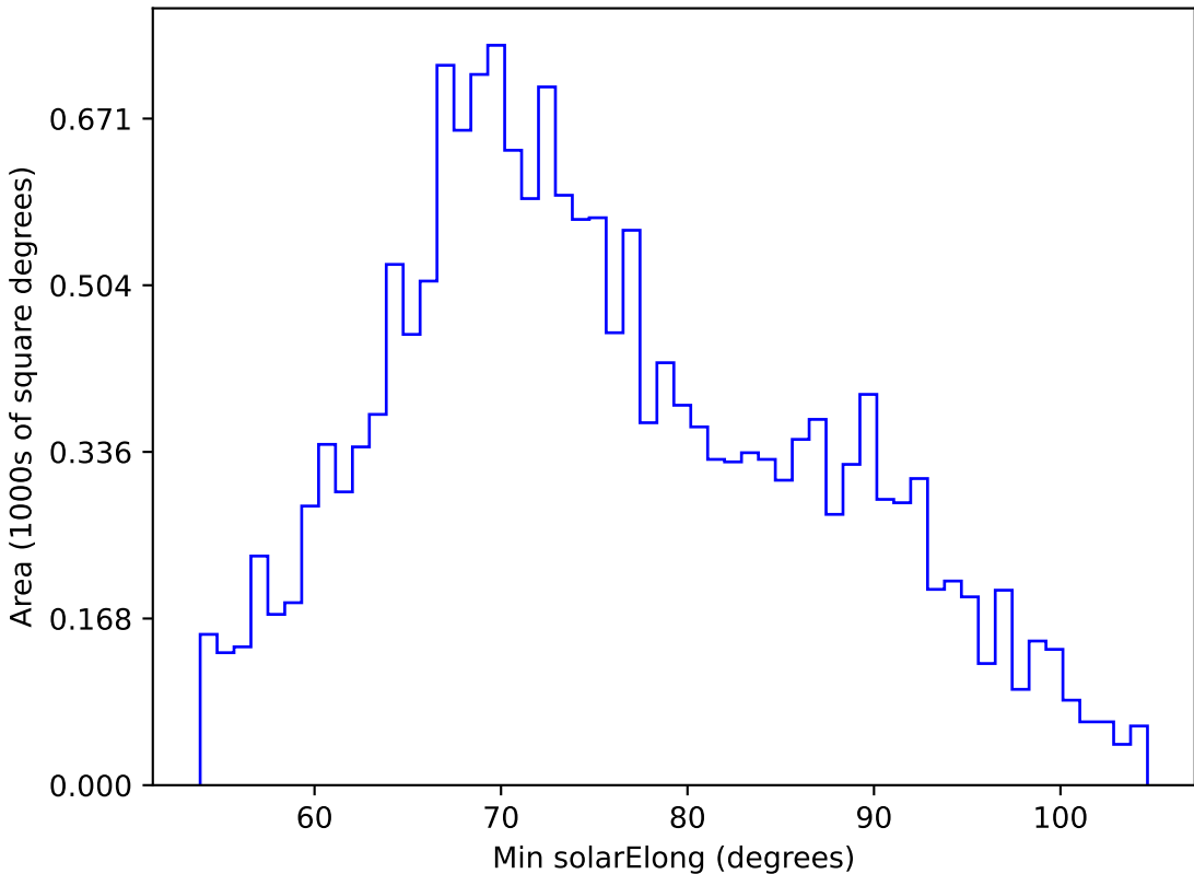
weather_cloudso18v3.4_10yrs WFD u band: Min solarElong
