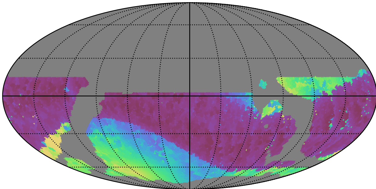
weather_cloudso18v3.4_10yrs WFD i band: Min solarElong
