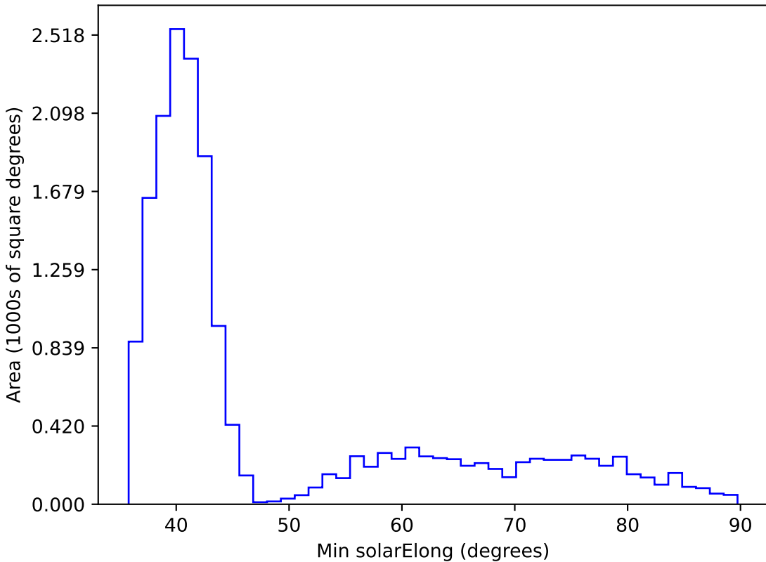
weather_cloudso18v3.4_10yrs WFD i band: Min solarElong
