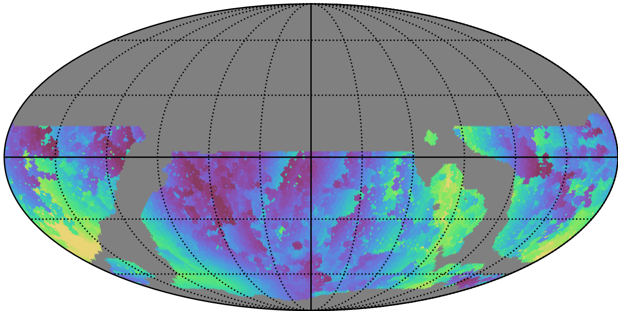
weather_cloudso18v3.4_10yrs WFD g band: Min solarElong
