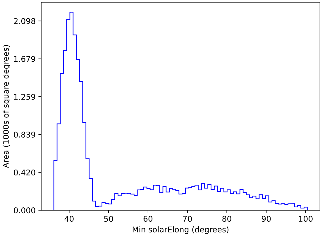
weather_cloudso18v3.4_10yrs All sky z band: Min solarElong
