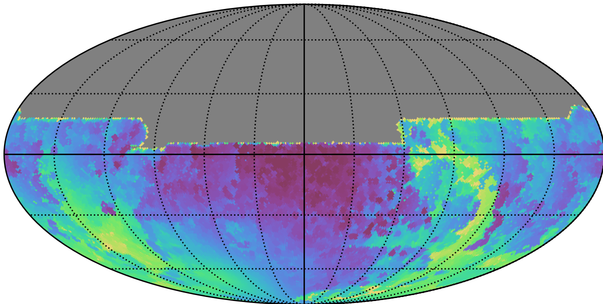
weather_cloudso18v3.4_10yrs All sky y band: Min solarElong
