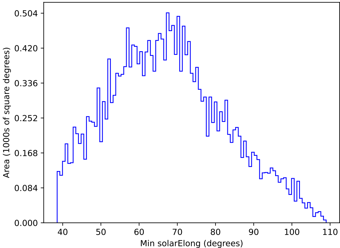
weather_cloudso18v3.4_10yrs All sky y band: Min solarElong
