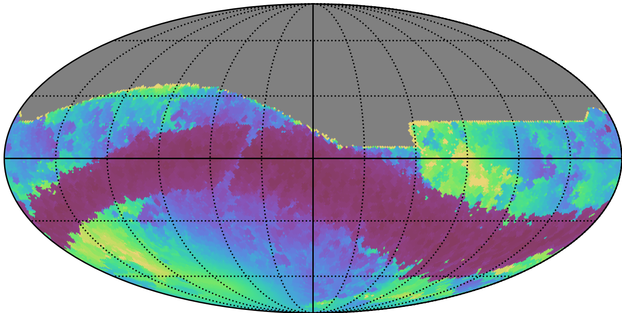
weather_cloudso18v3.4_10yrs All sky r band: Min solarElong
