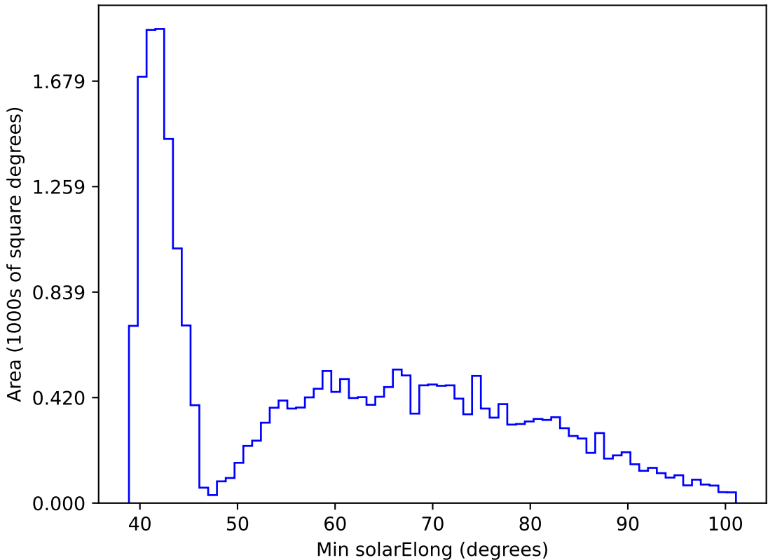
weather_cloudso18v3.4_10yrs All sky r band: Min solarElong
