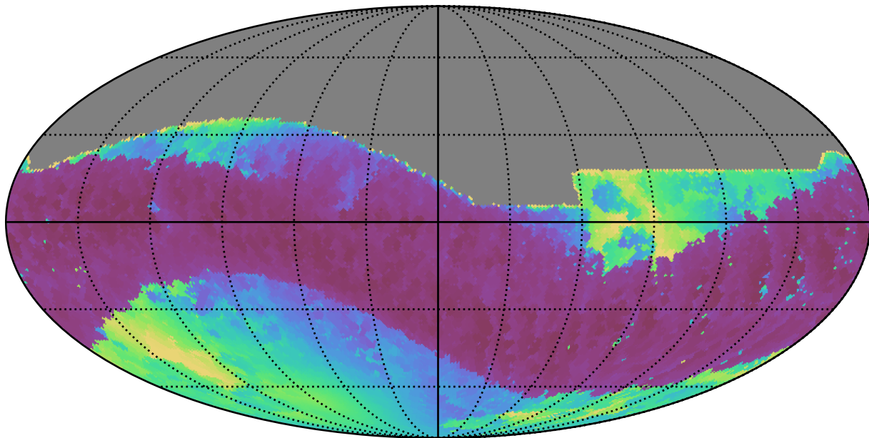
weather_cloudso18v3.4_10yrs All sky i band: Min solarElong
