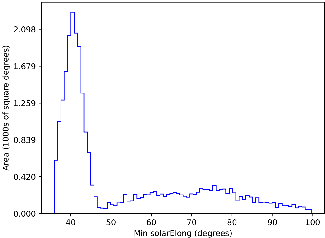
weather_cloudso18v3.4_10yrs All sky i band: Min solarElong
