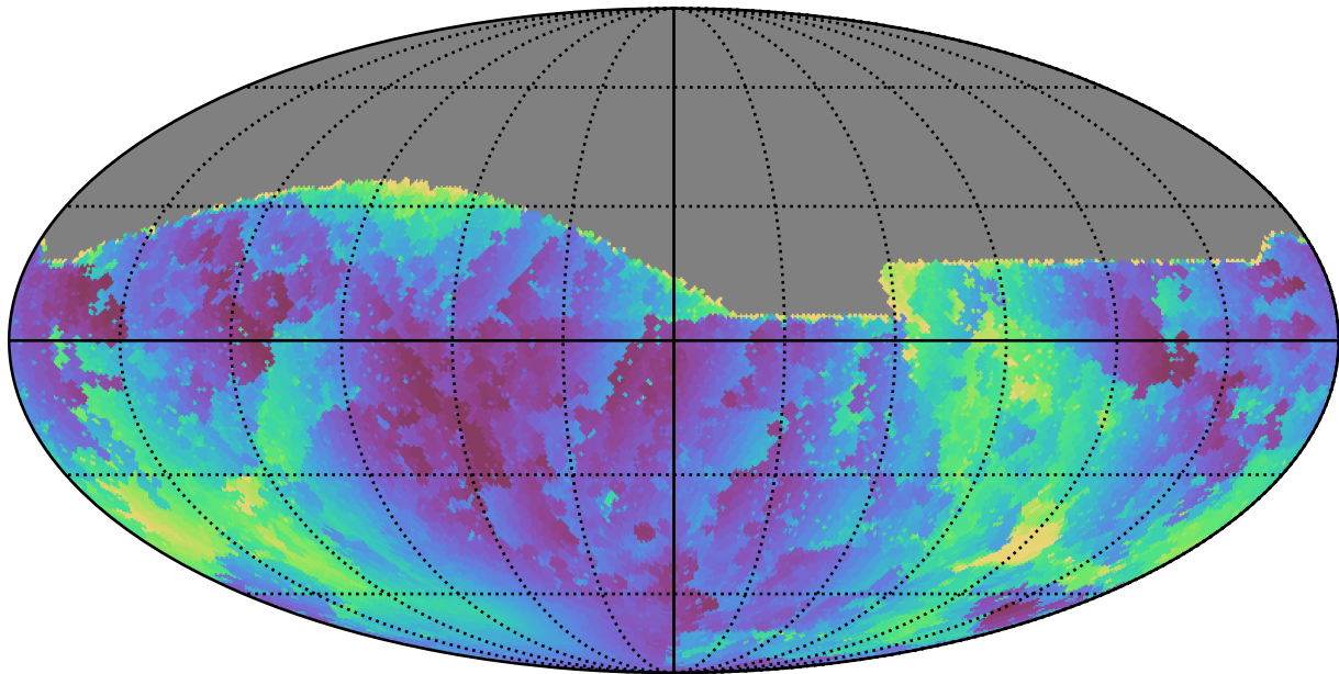
weather_cloudso18v3.4_10yrs All sky g band: Min solarElong
