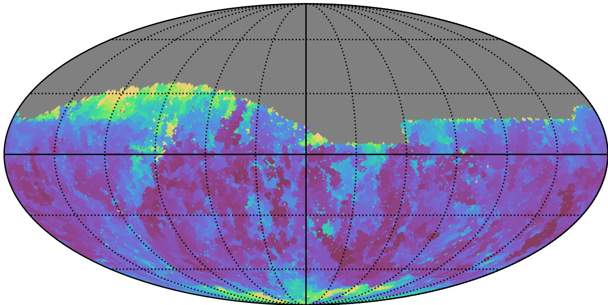
weather_cloudso18v3.4_10yrs Yr 1 z band: Min seeingGeom
