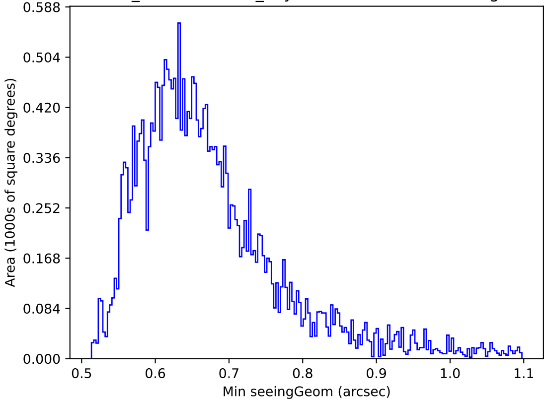
weather_cloudso18v3.4_10yrs Yr 1 z band: Min seeingGeom
